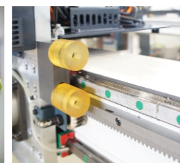
X轴限位位置弹性防撞块
